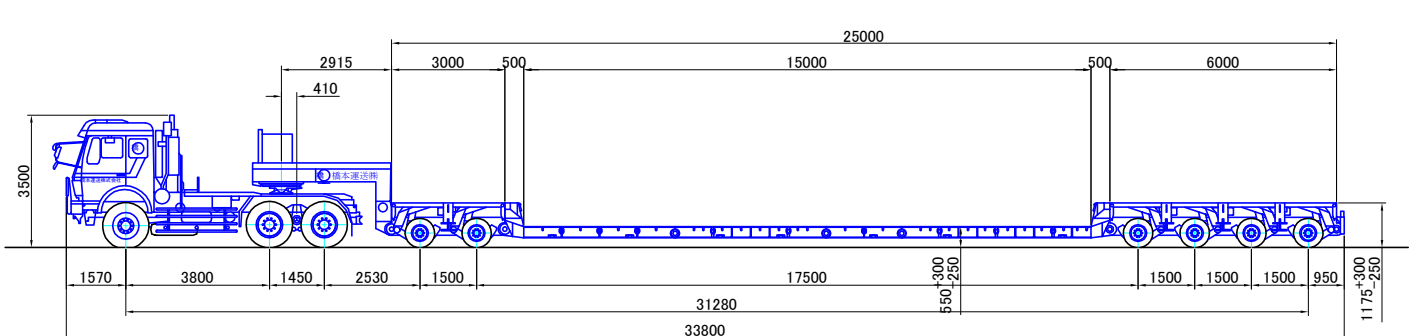
6軸バージョン (Version 35) 最大積載量 170,000kg (構内最大 180.38トン)
