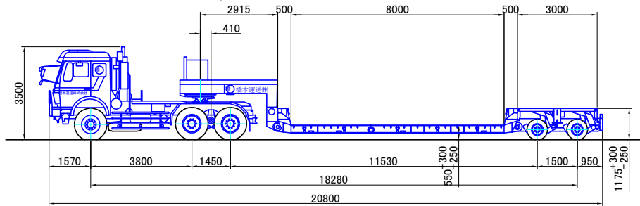
2軸バージョン (Version 32) 最大積載量 66,000kg (構内最大 81.10ト)
