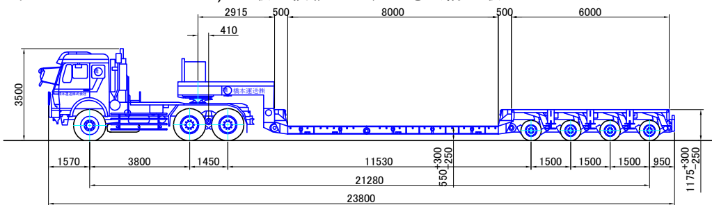
4軸バージョン (Version 34) 最大積載量 85,000kg (構内最大 142.50ト)
