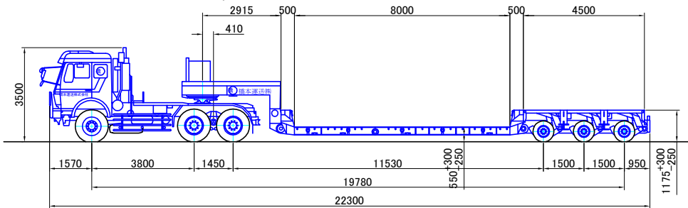
3軸バージョン (Version 33) 最大積載量 85,000kg (構内最大 111.80ト)
