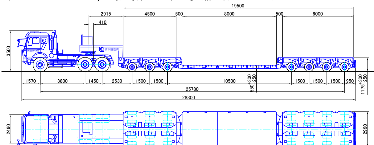
7軸バージョン (Version 36) 最大積載量 170,000kg (構内最大 221.90ト)
