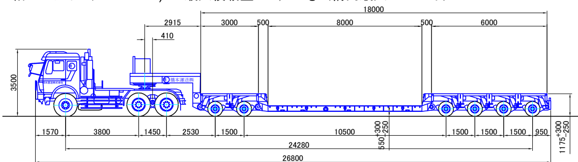
6軸バージョン (Version 35) 最大積載量 170,000kg (構内最大 191.15ト)
