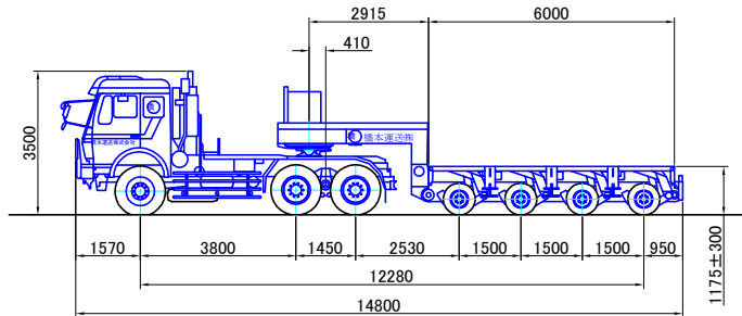
4軸バージョン (Version 11) 最大積載量 85,000kg (構内最大 147.80ト)
