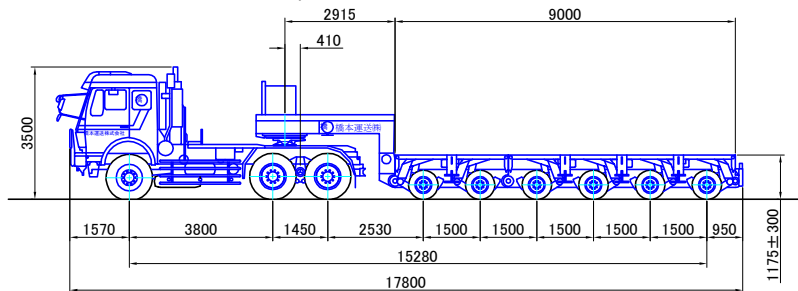
6軸バージョン (Version 3) 最大積載量 170,000kg (構内最大 206.45ト)
