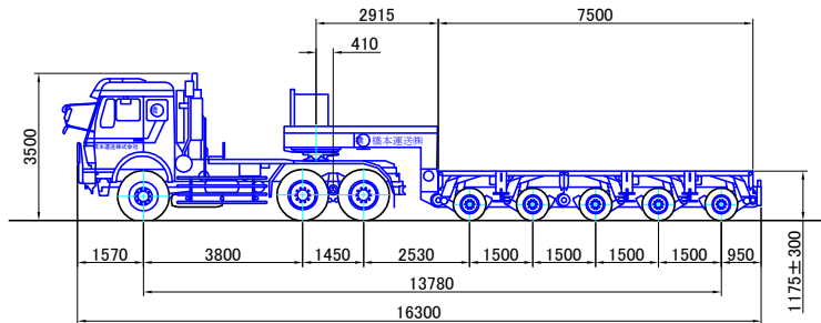
5軸バージョン (Version 25) 最大積載量 85,000kg (構内最大 175.75ト)
