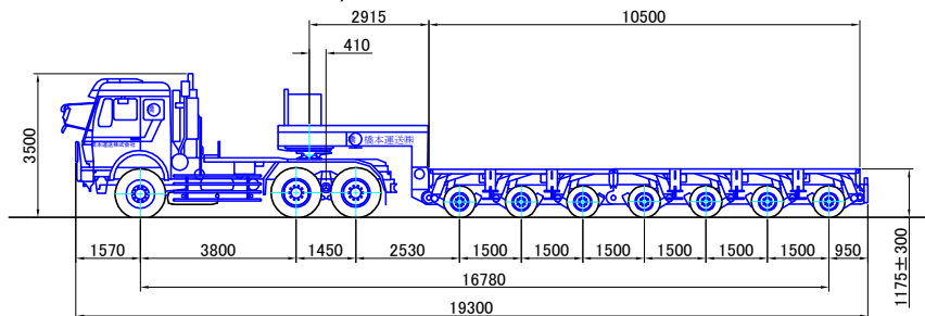
7軸バージョン (Version 20) 最大積載量 170,000kg (構内最大 236.65ト)
