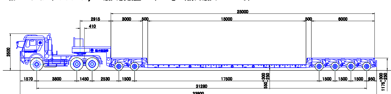
6軸バージョン (Version 35) 最大積載量 170,000kg (構内最大 180.38 t )
