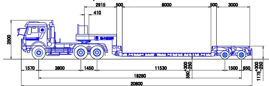
2軸バージョン (Version 32) 最大積載量 66,000kg (構内最大 81.10トﾝ)
