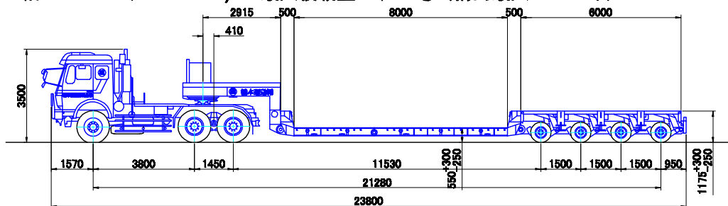
4軸バージョン (Version 34) 最大積載量 85,000kg (構内最大 142.50トﾝ)
