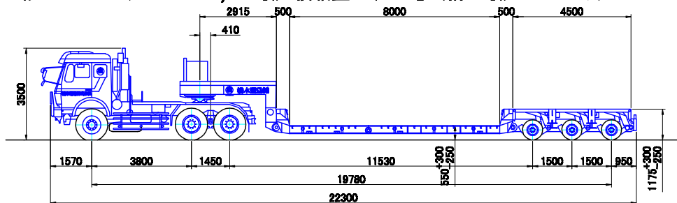
3軸バージョン (Version 33) 最大積載量 85,000kg (構内最大 111.80トﾝ)
