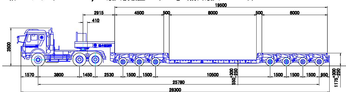
7軸バージョン (Version 36) 最大積載量 170,000kg (構内最大 221.90トﾝ)
