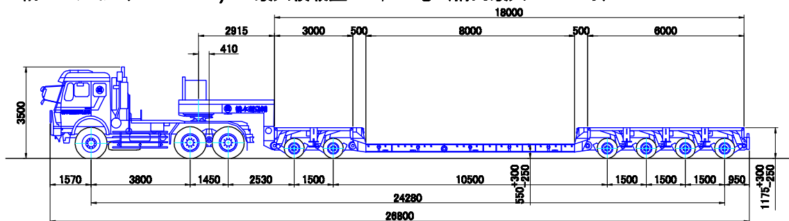
6軸バージョン (Version 35) 最大積載量 170,000kg (構内最大 191.15トﾝ)
