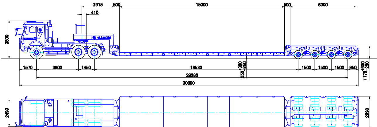
4軸バージョン (Version 34) 最大積載量 85,000kg (構内最大 125.02ト)
